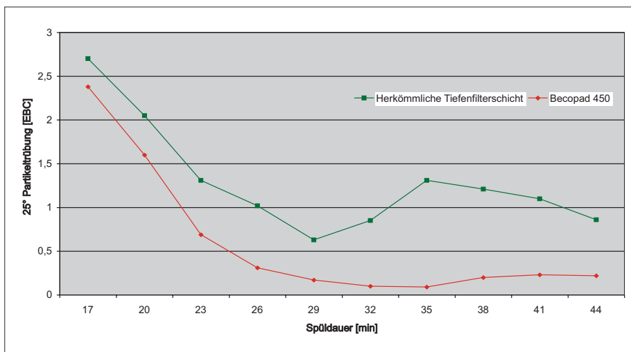
Abb. 2: Verlauf der Partikeltrübung im Spülwasser
