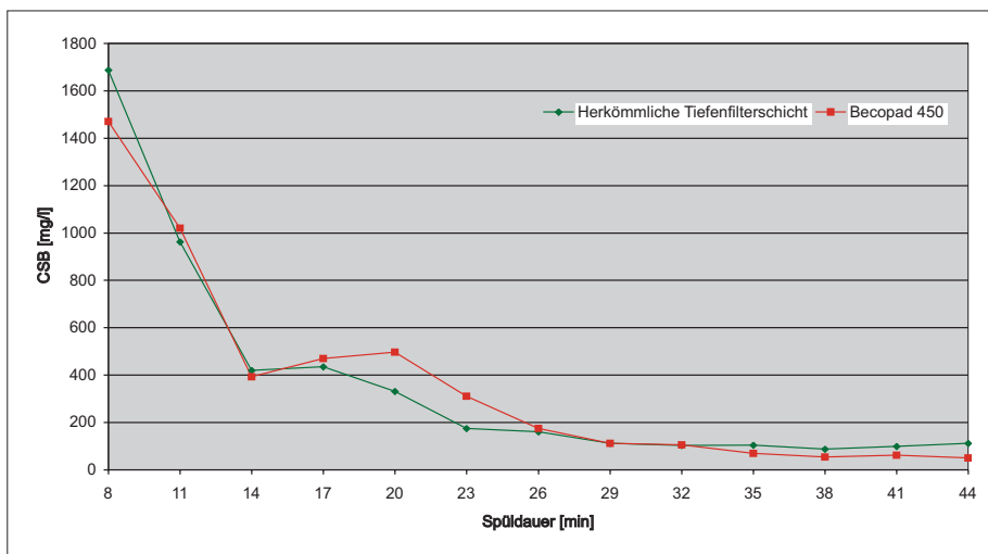
Abb. 1: Verlauf der CSB-Werte im Spülwasser
